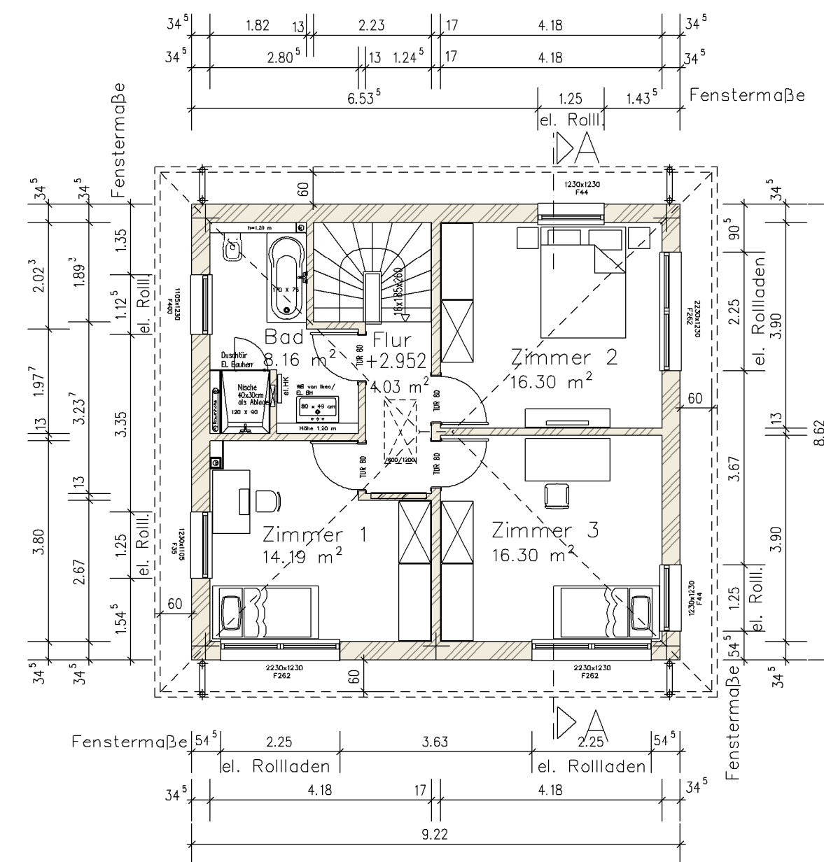
Obergeschoss
