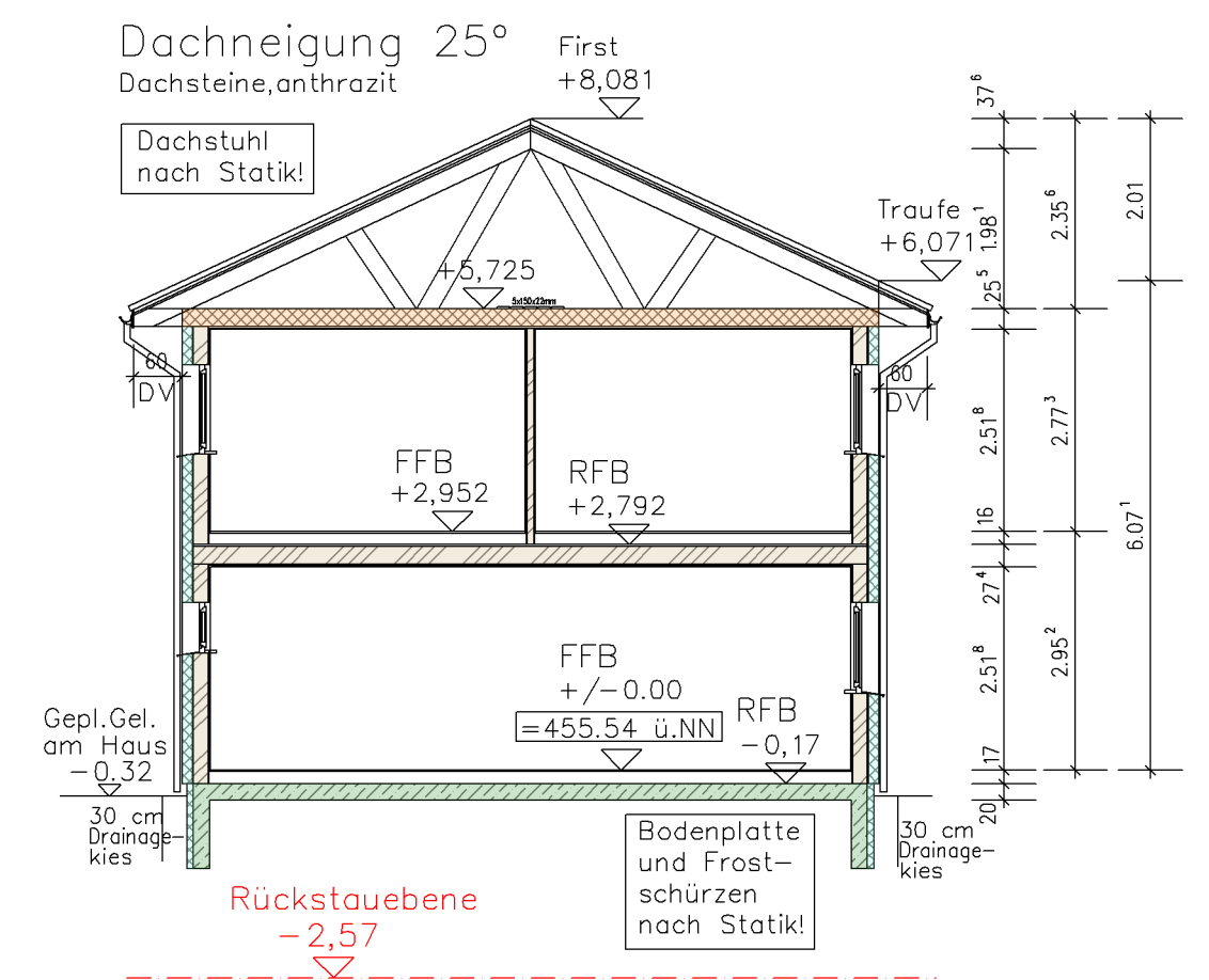
Schnitt A-A (Wohnhaus)
