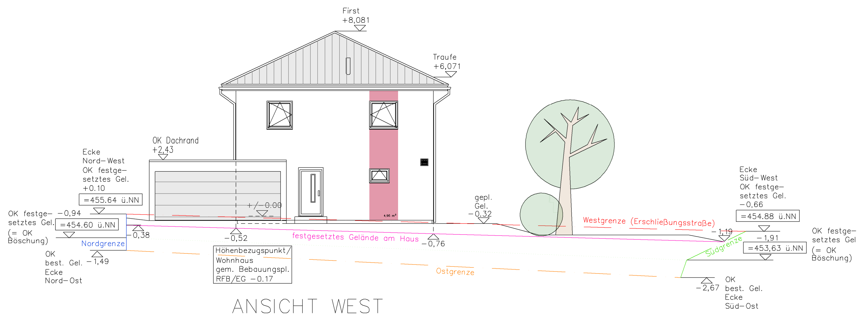
Ansicht West
