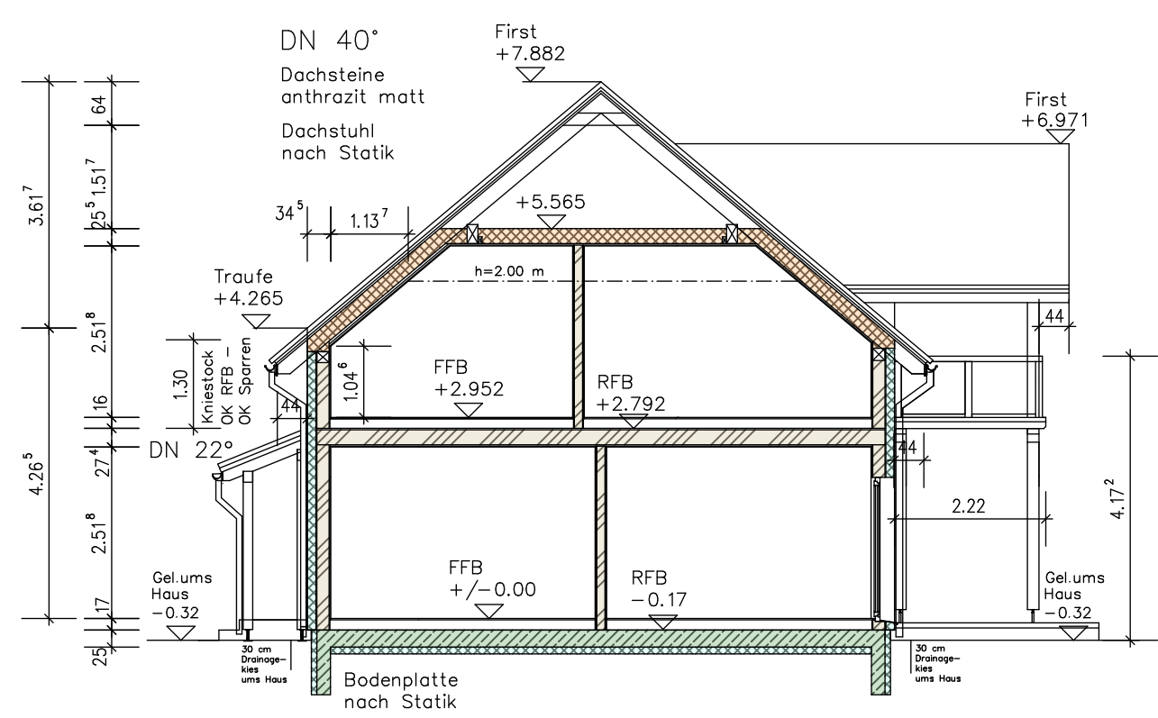
Schnitt A-A (Wohnhaus)
