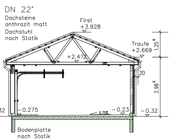
Schnitt Garage
