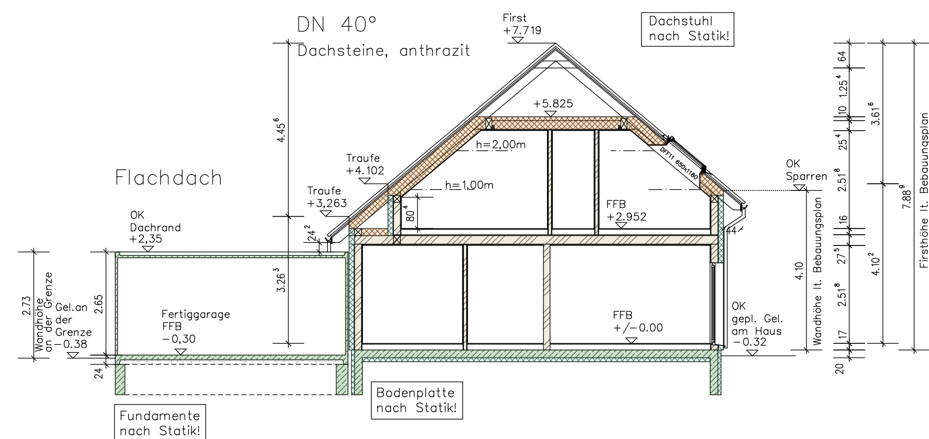
Schnitt A-A
