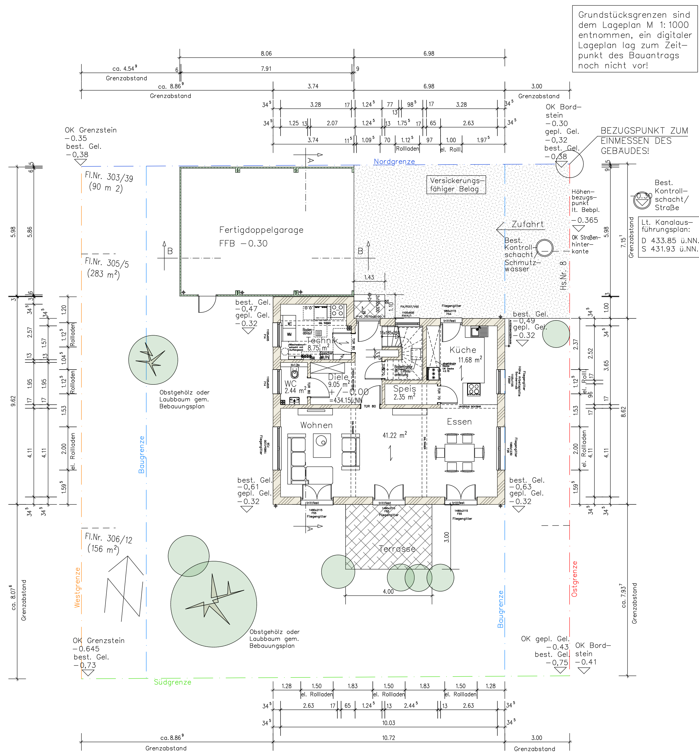
Erdgeschoss
