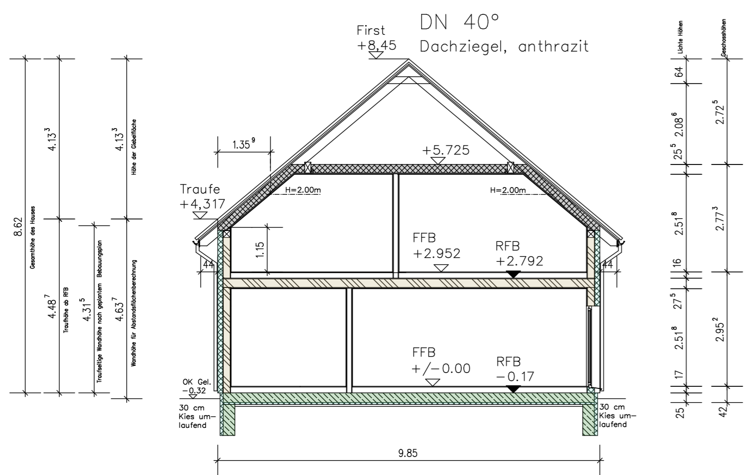
SCHNITT A-A
