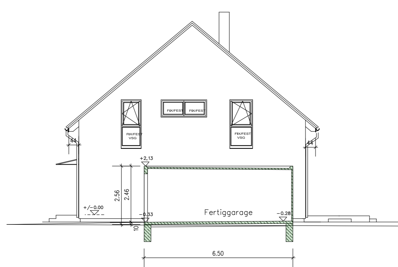
SCHNITT B-B
