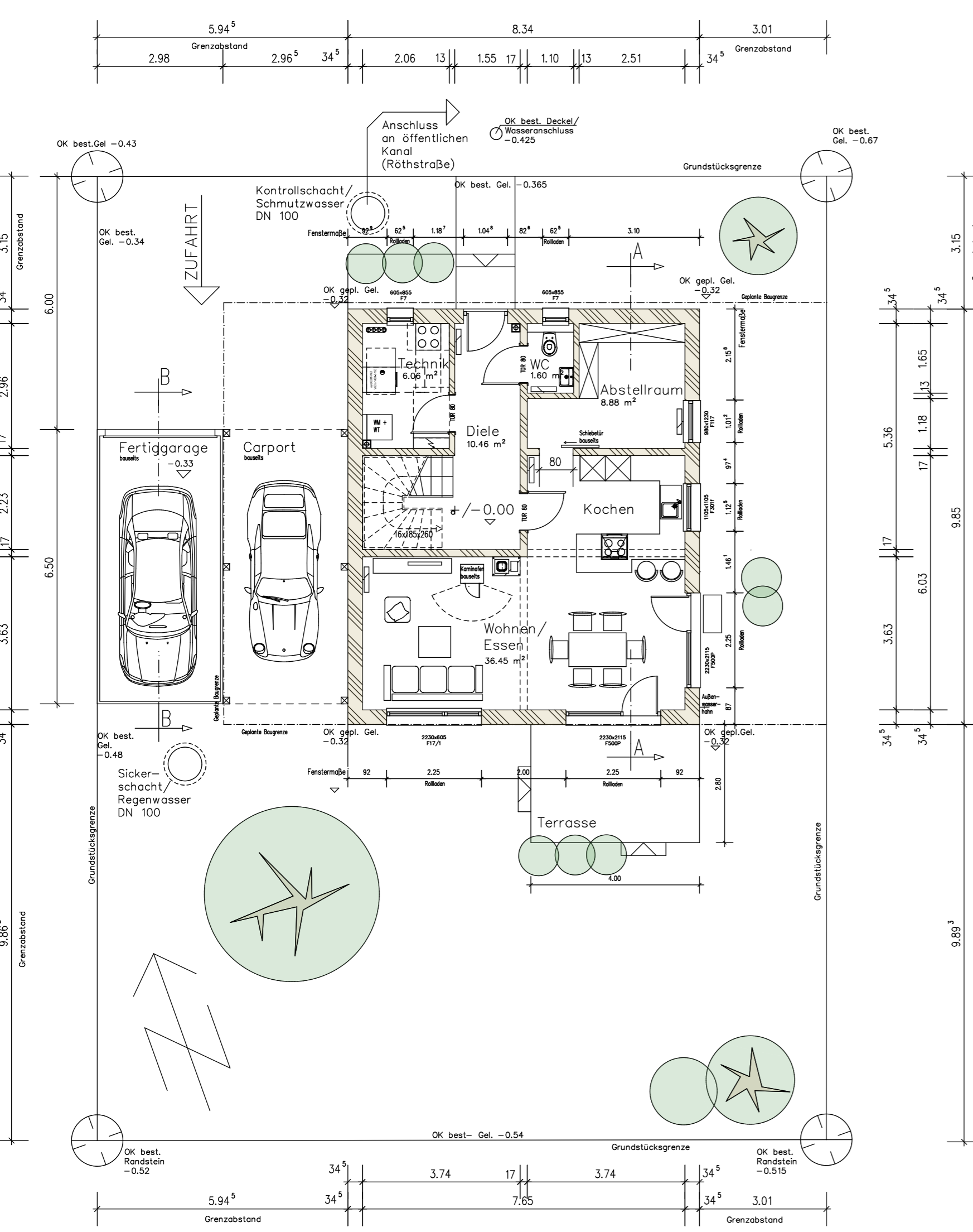
ERDGESCHOSS
