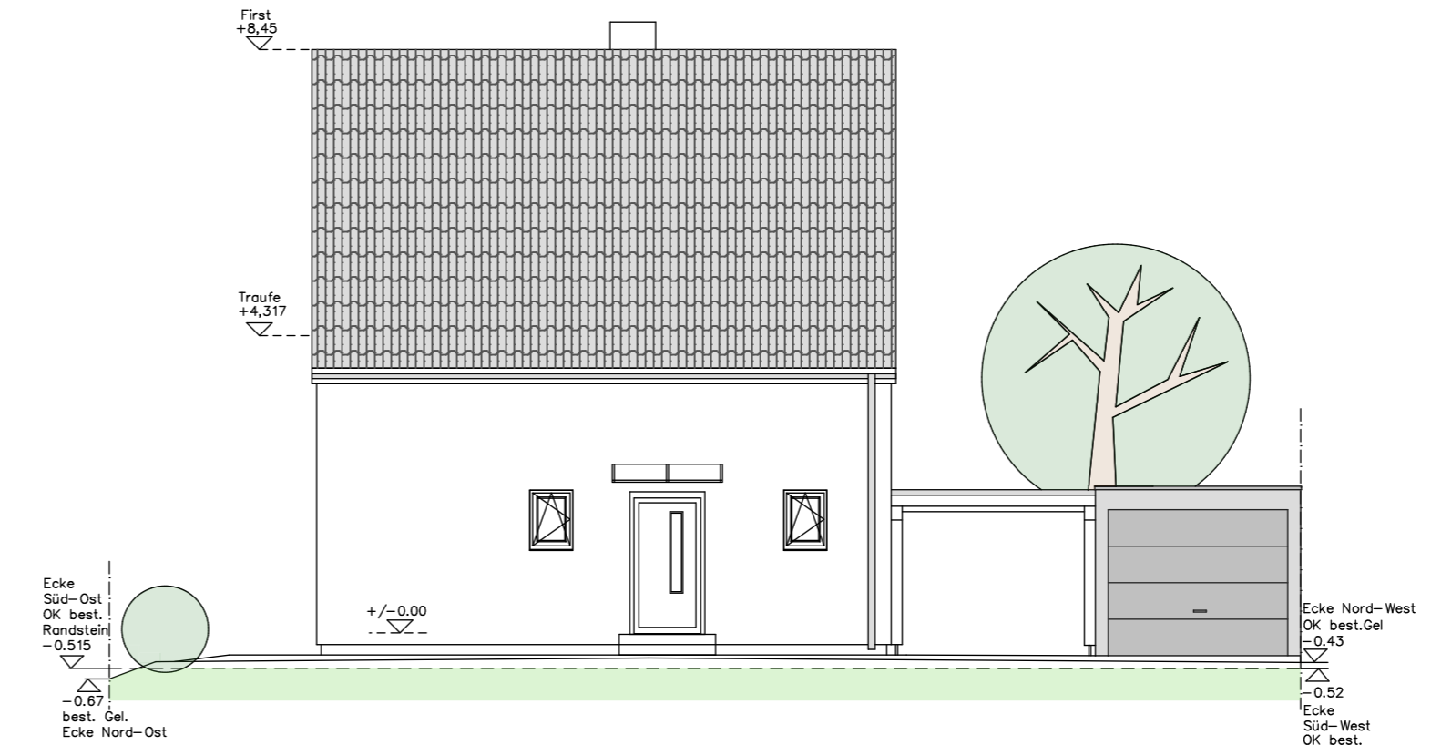
ANSICHT NORDEN
