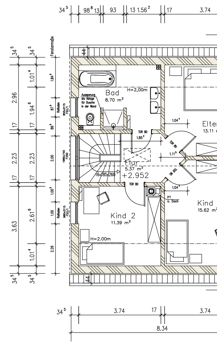
DACHGESCHOSS
