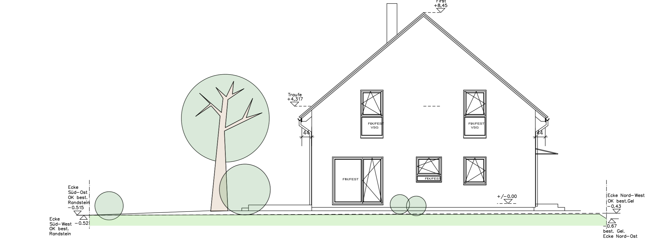
ANSICHT OSTEN
