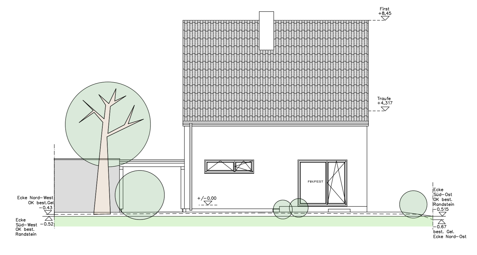
ANSICHT SÜDEN
