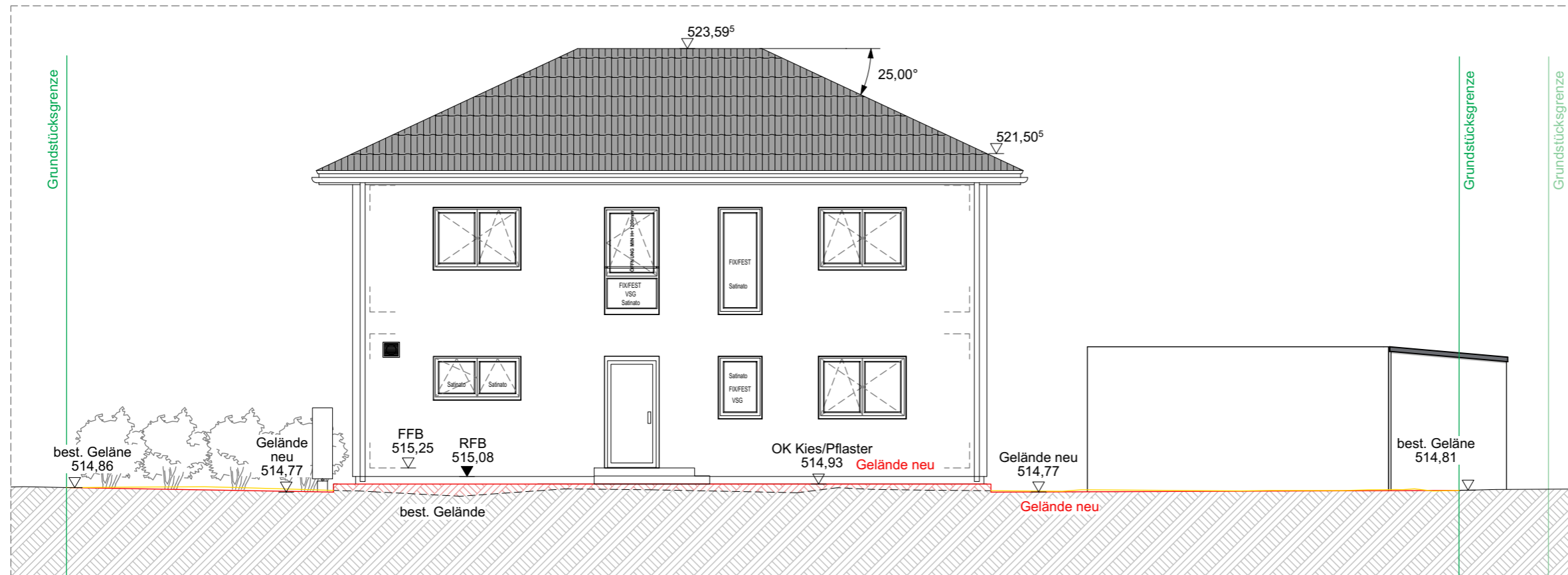
Ansicht Nord
