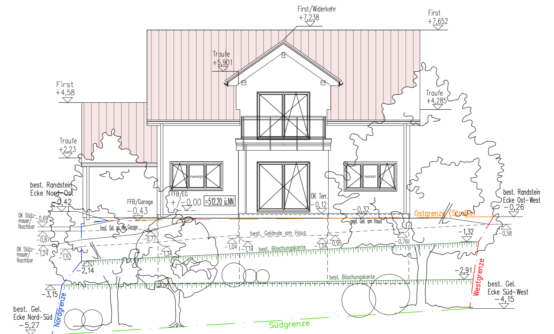
Ansicht West
