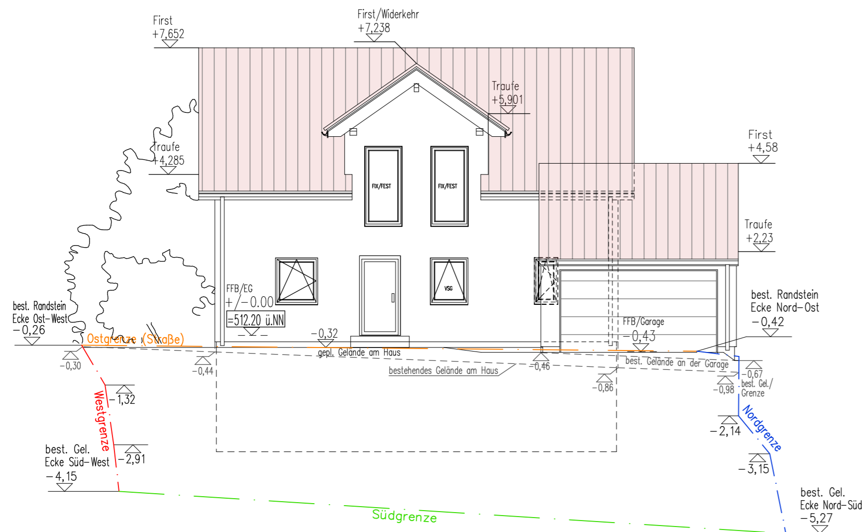
Ansicht Ost
