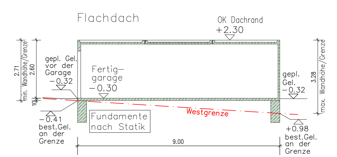
Schnitt B-B
