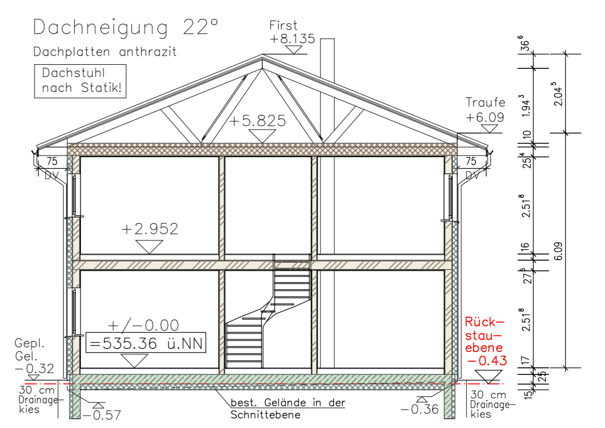
Schnitt A-A
