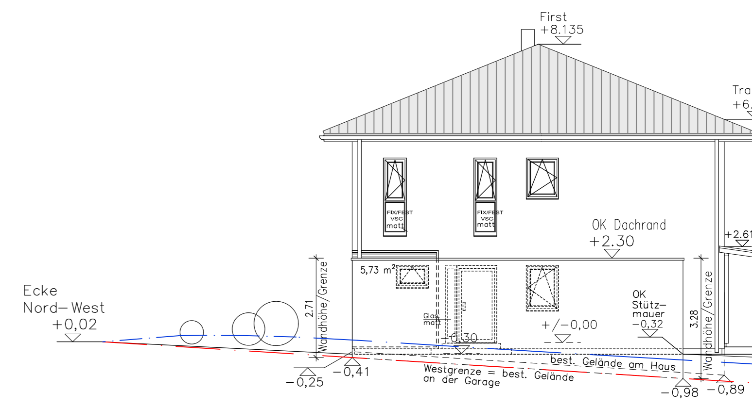
Ansicht West
