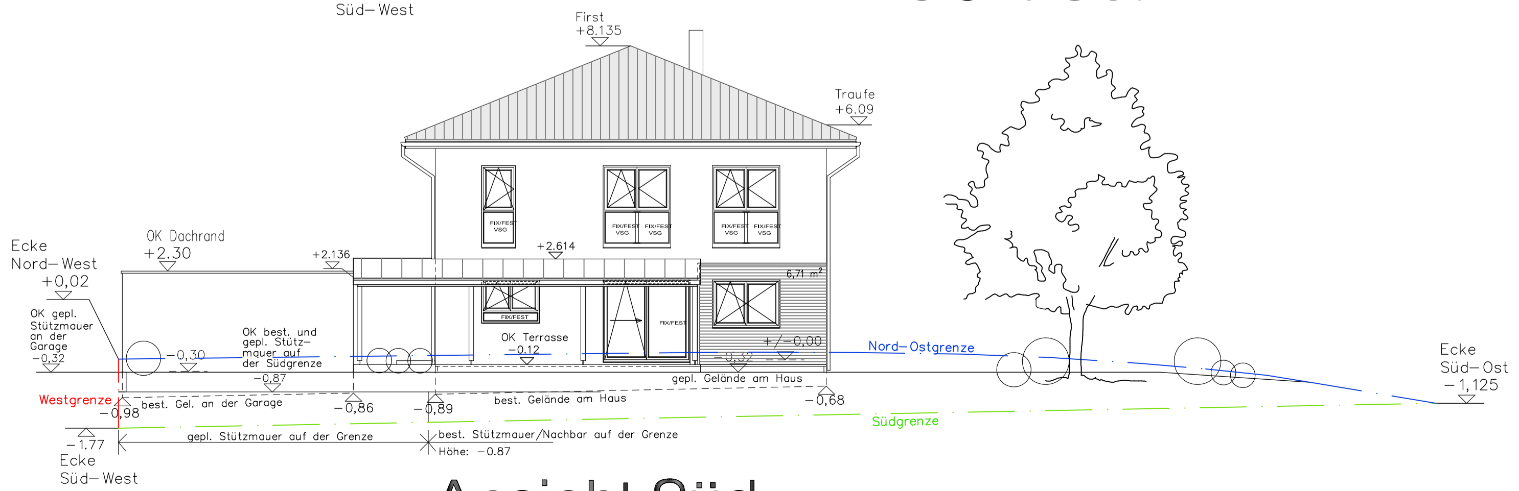
Ansicht Ost
