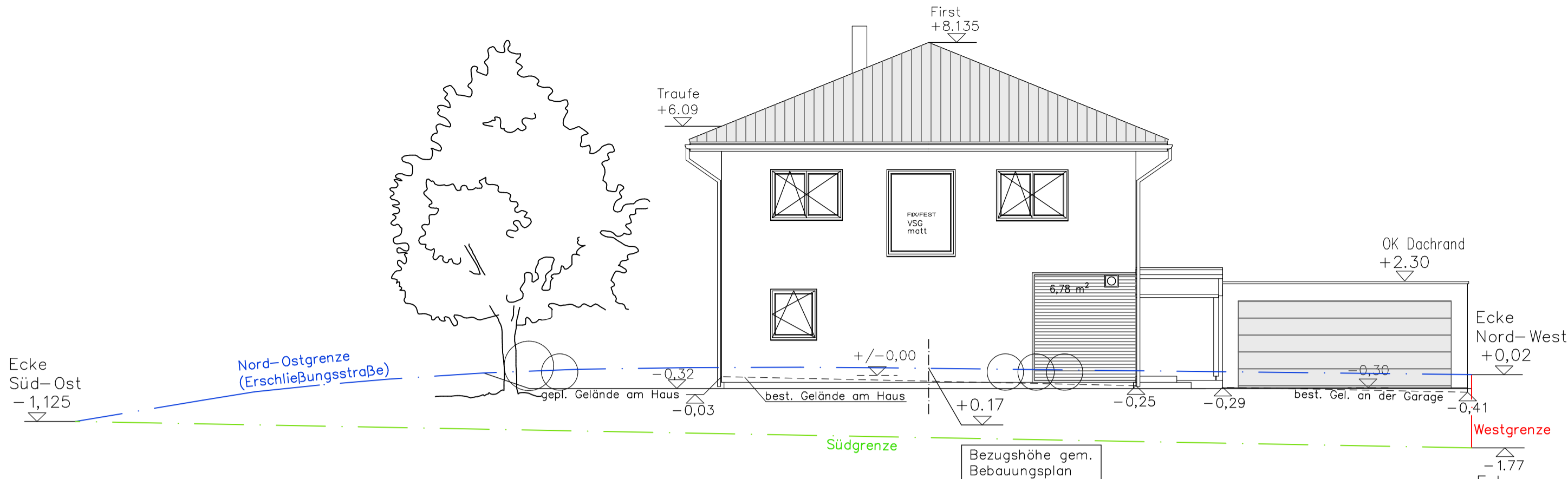
Ansicht Nord
