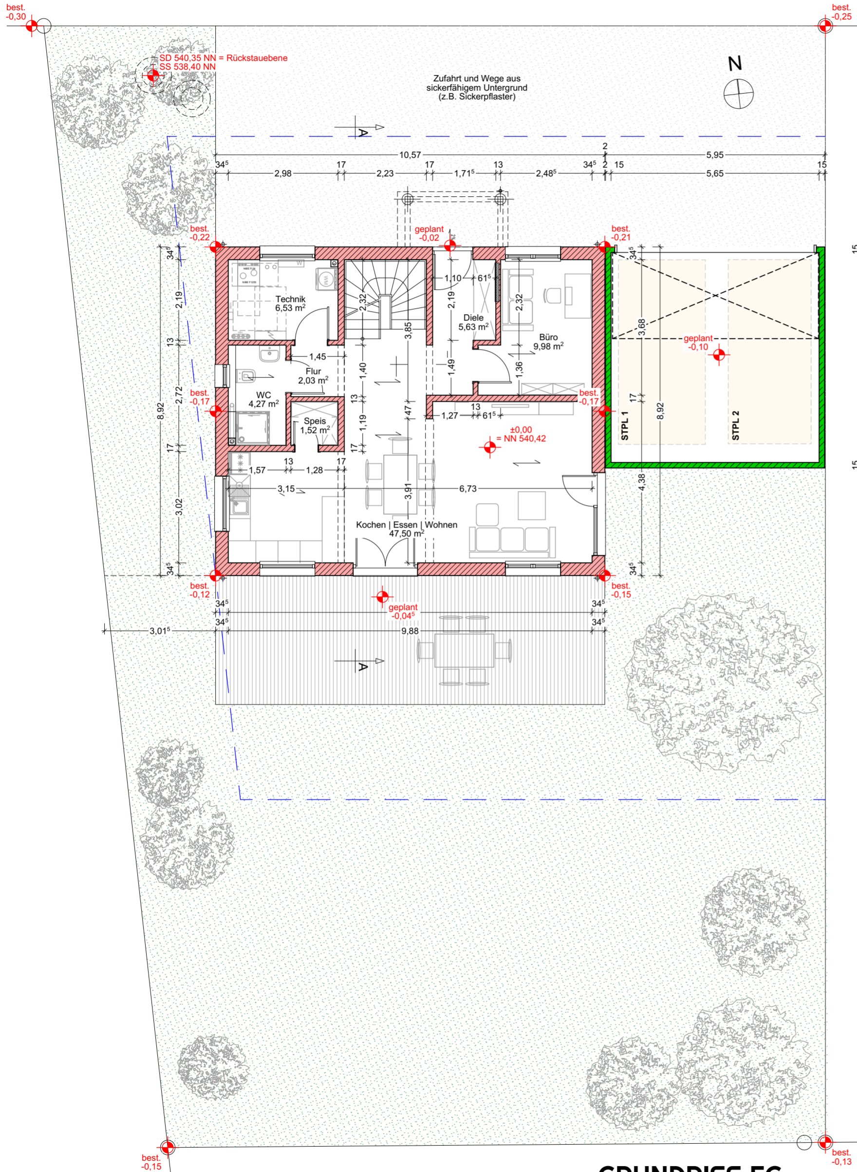
GRUNDRISS EG
