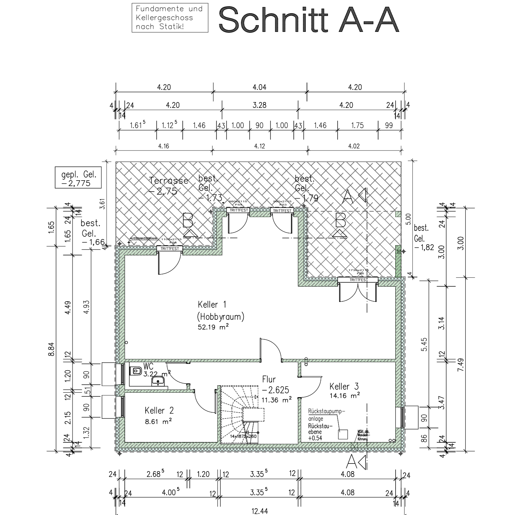
Kellergeschoß
