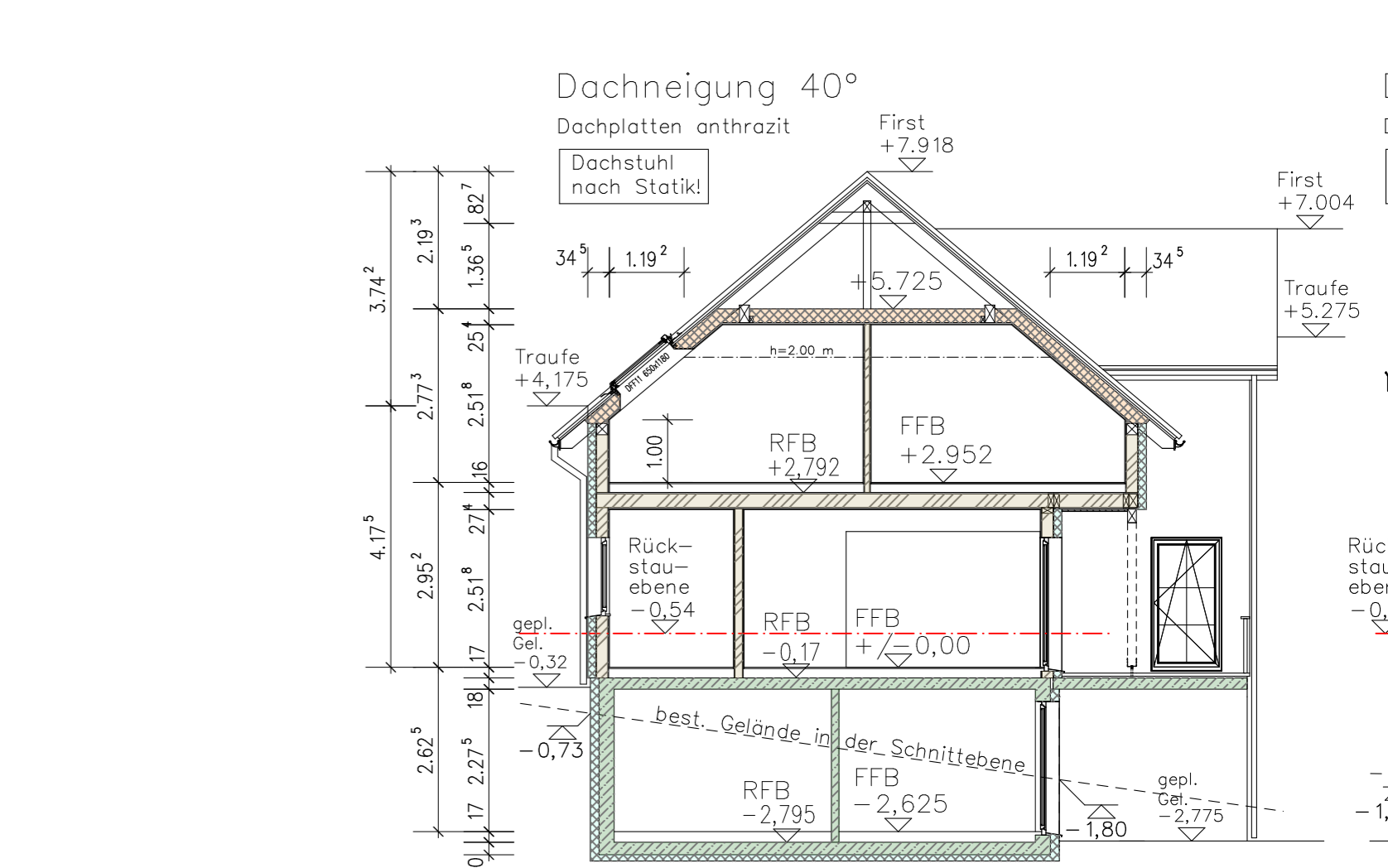
Schnitt A-A
