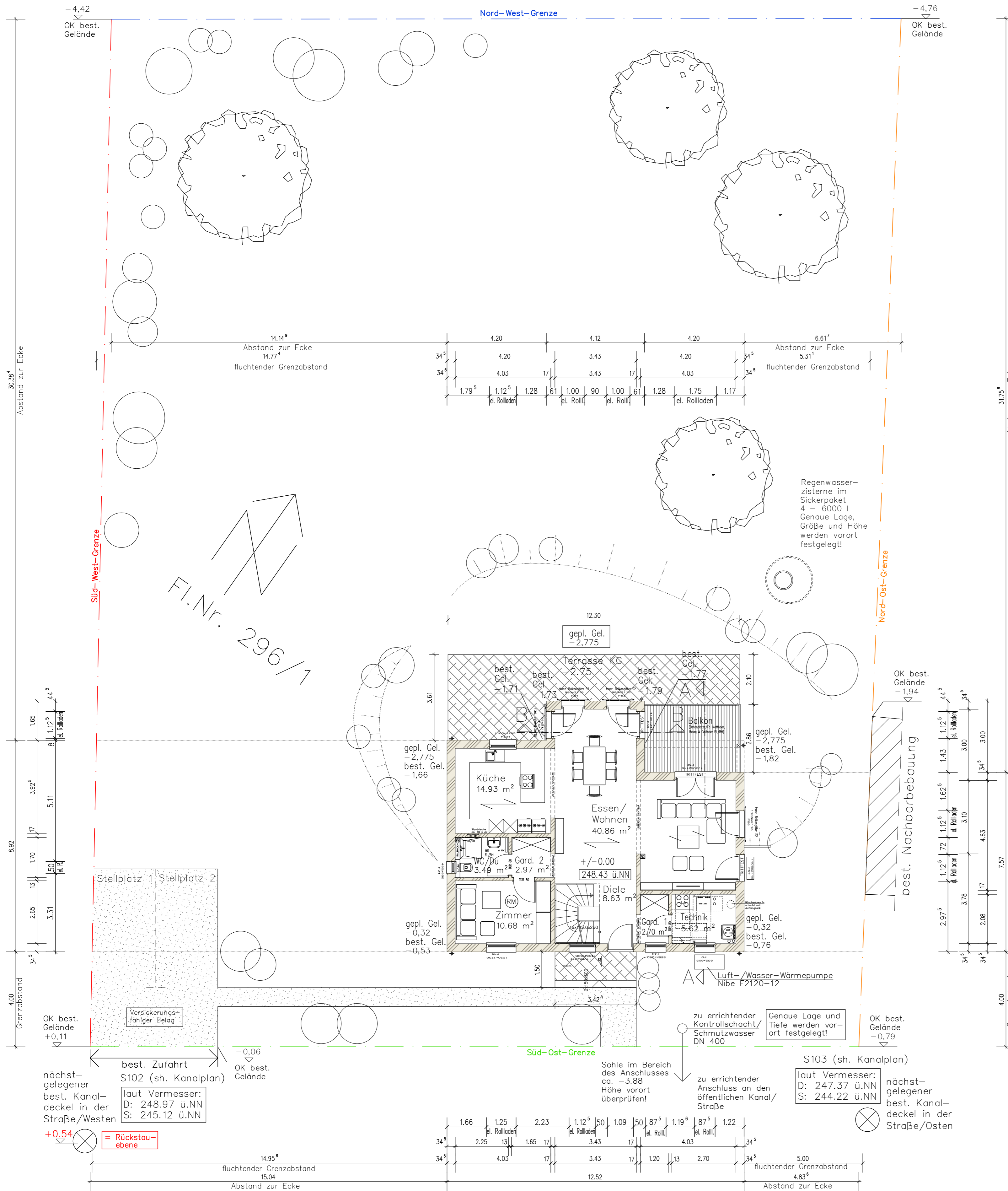
Erdgeschoss
