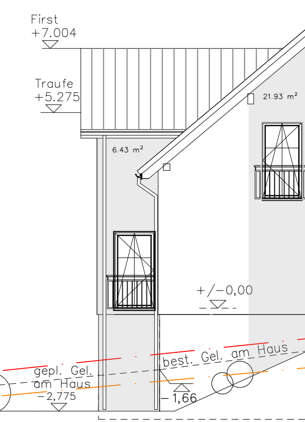
Ansicht
