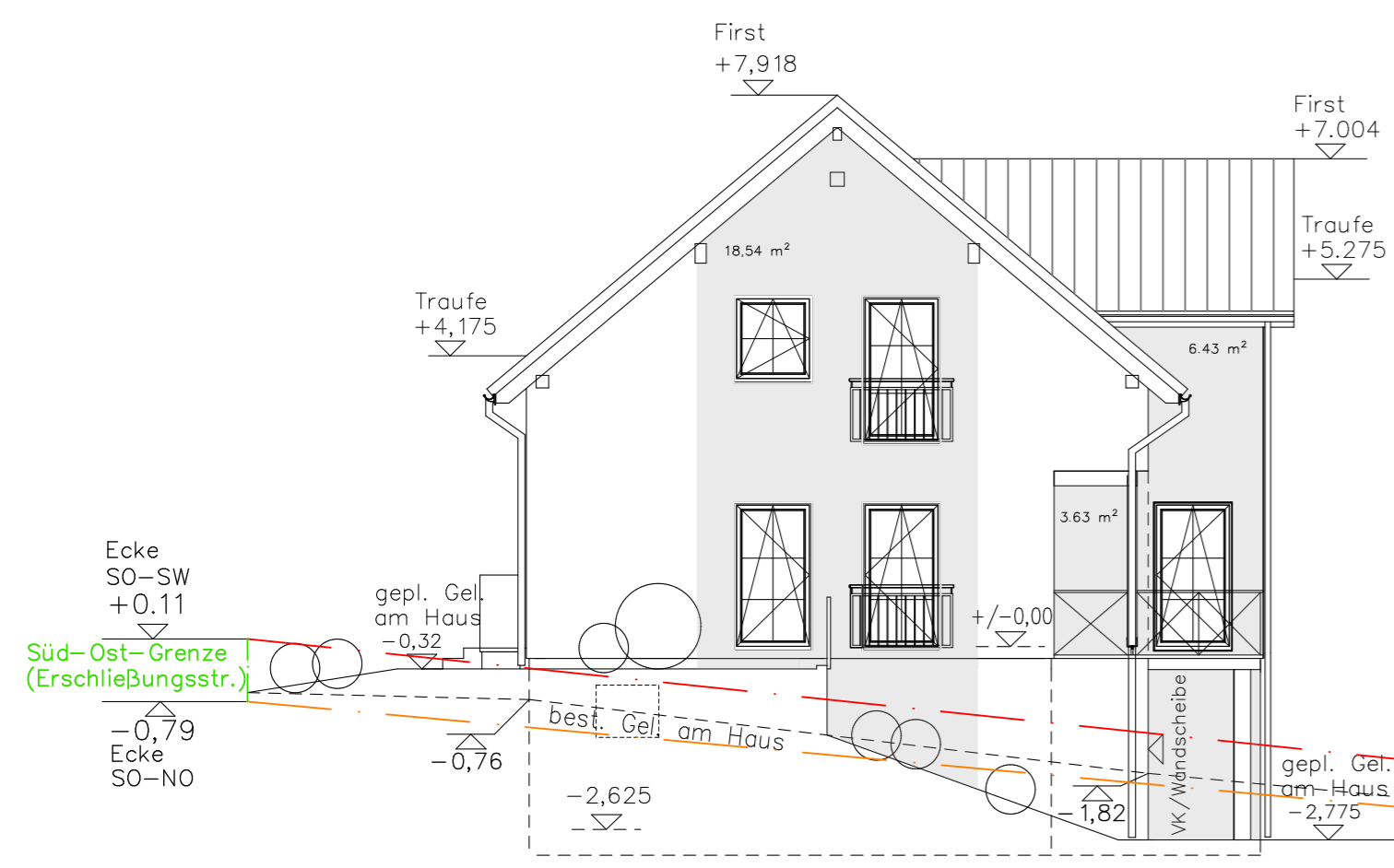
Ansicht Nord-Ost
