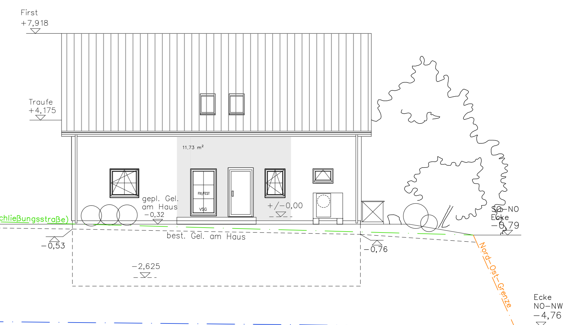
Ansicht Süd-Ost
