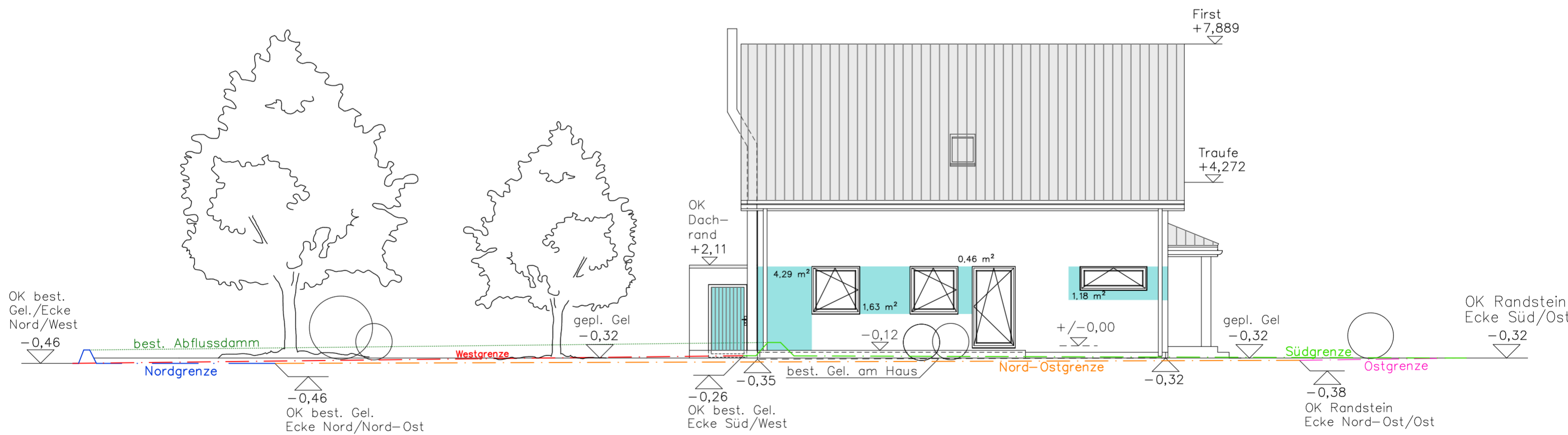
Ansicht Süd-West
