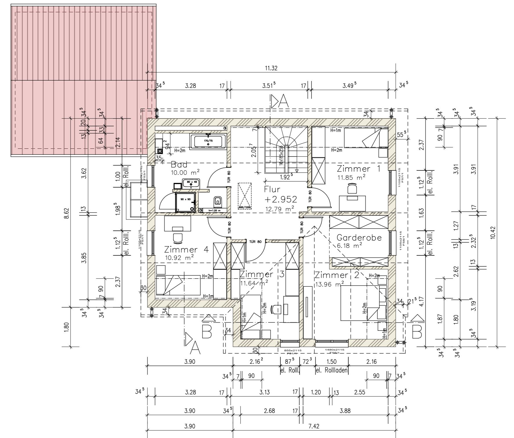
Dachgeschoss
