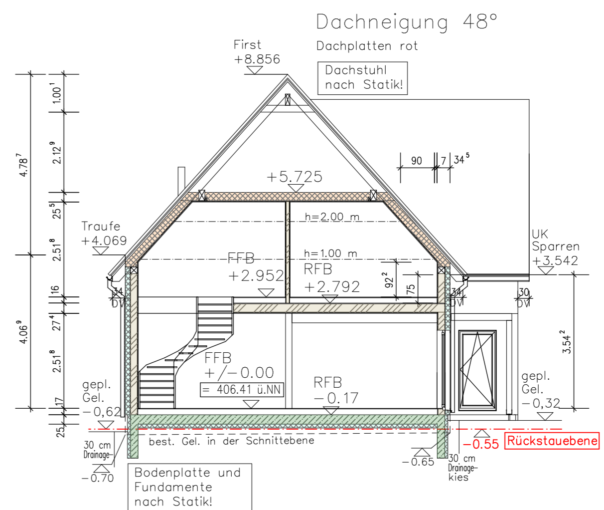
Schnitt A-A
