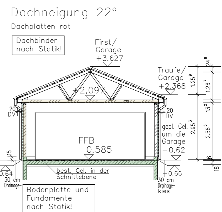
Schnitt C-C
