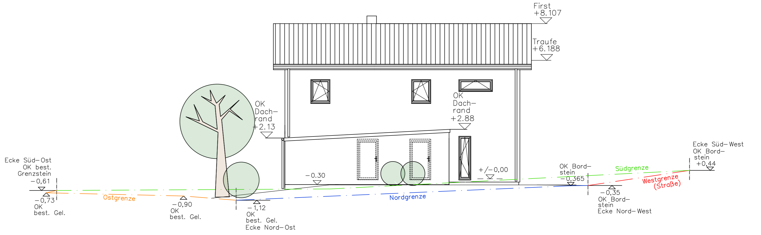
Ansicht Nord
