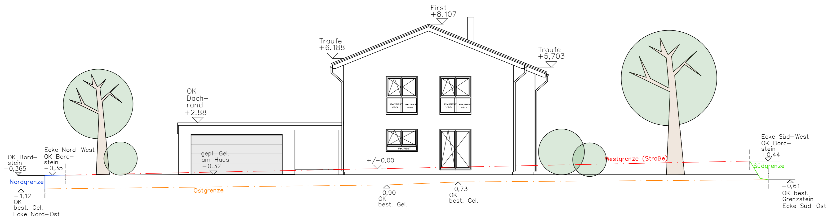
Ansicht West
