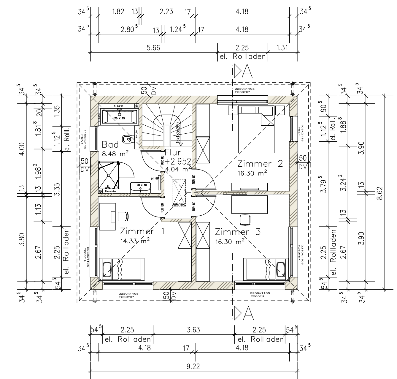
Obergeschoss
