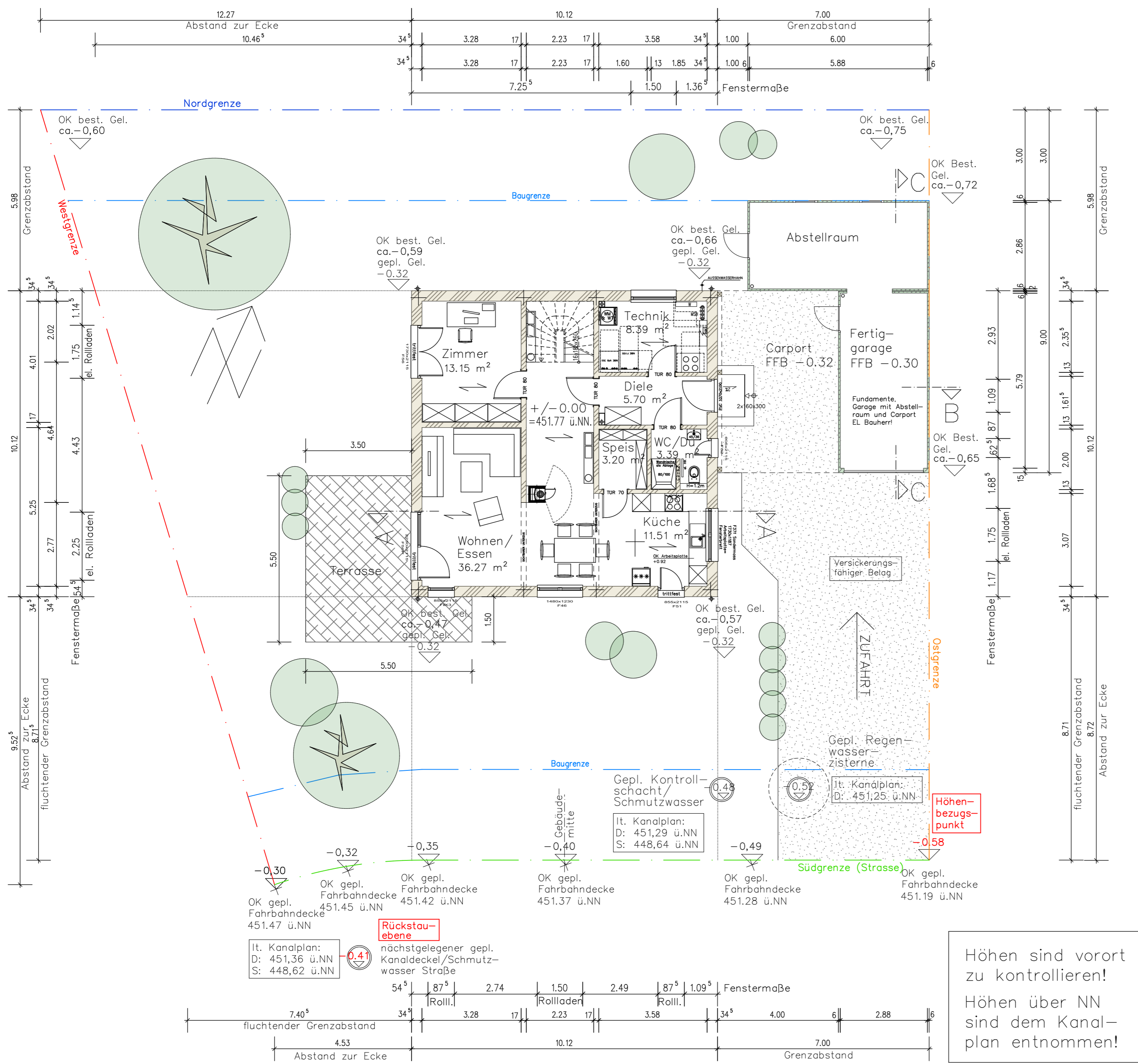
Erdgeschoss
