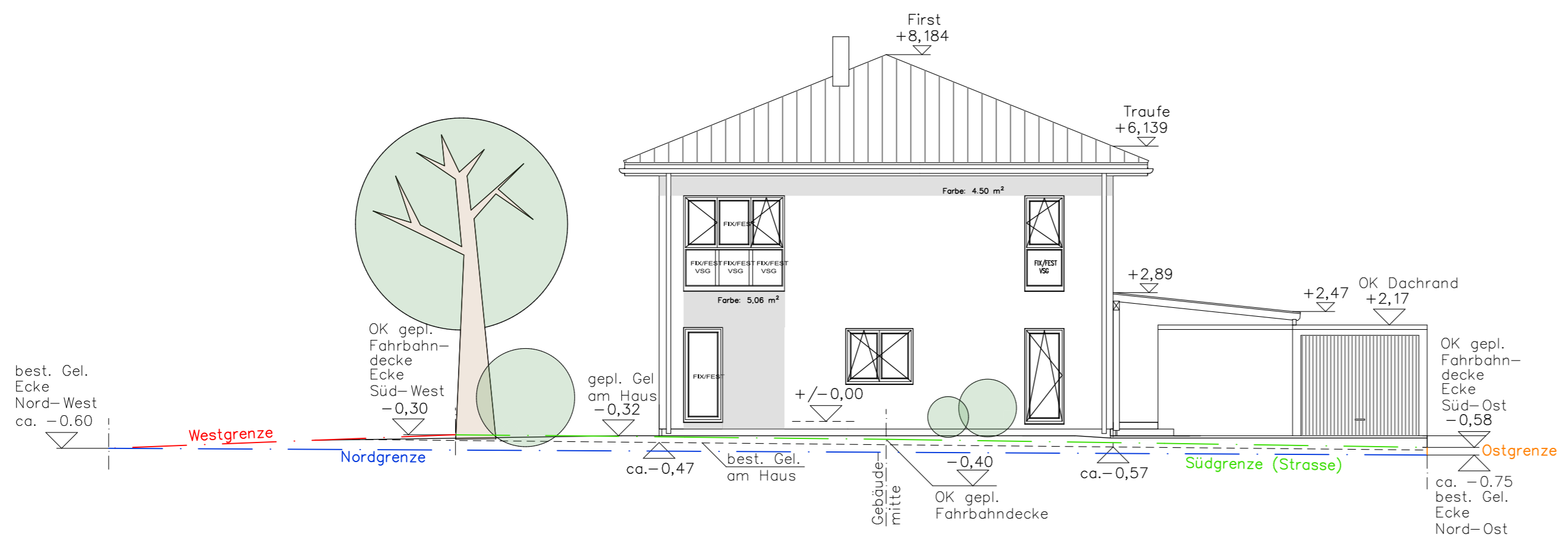
Ansicht Süd (Strasse)
