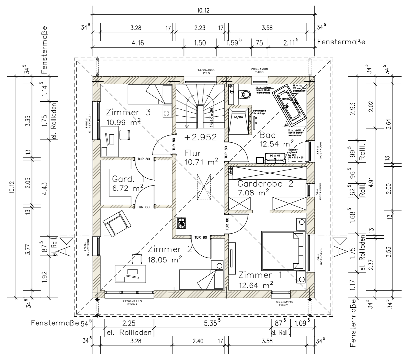
Obergeschoss
