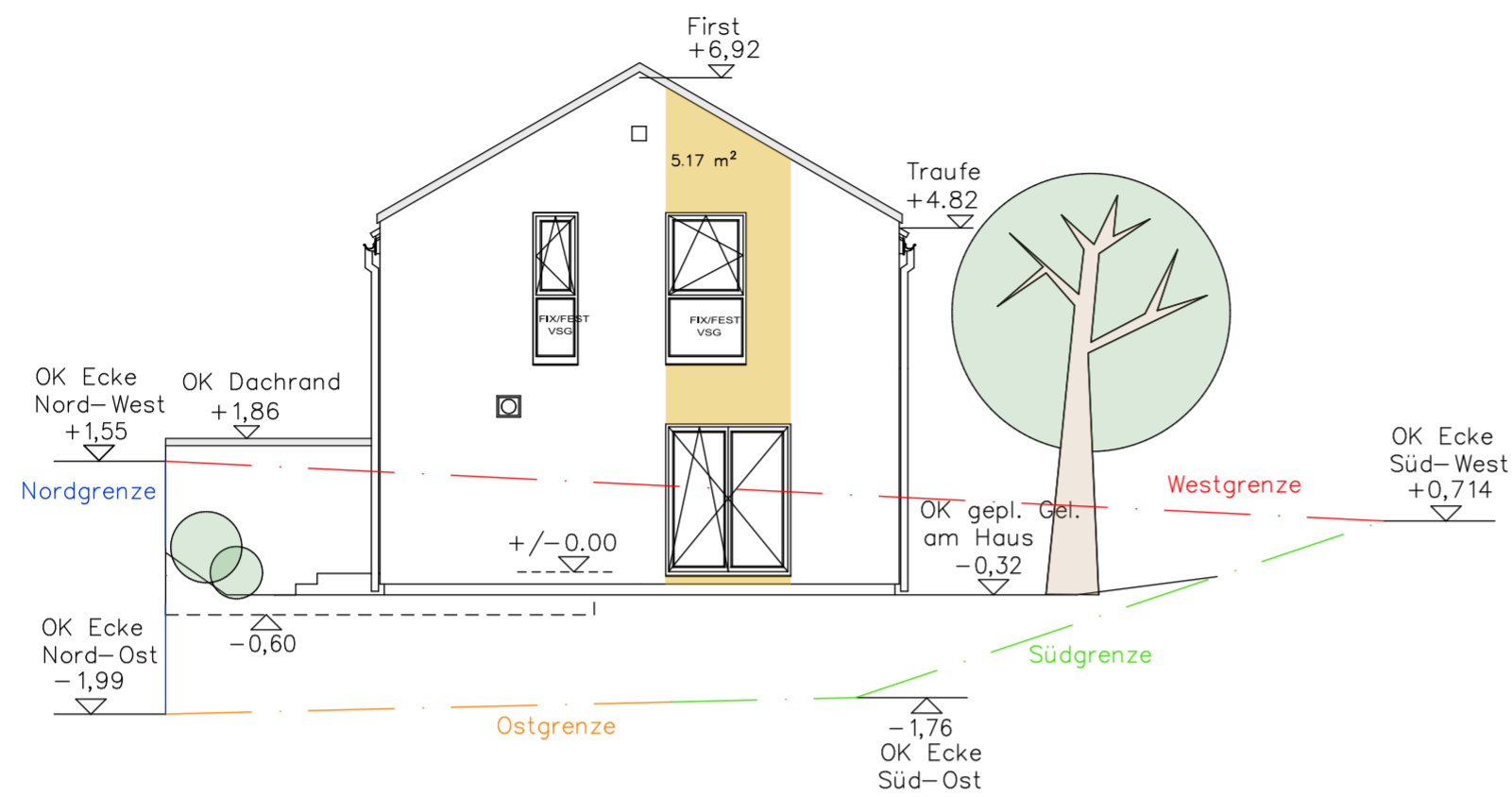
ANSICHT WEST
