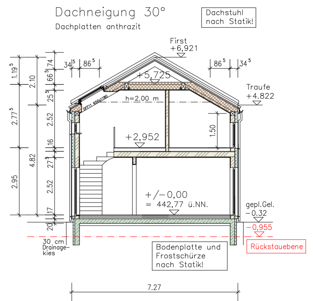
SCHNITT A-A (WOHNHAUS)
