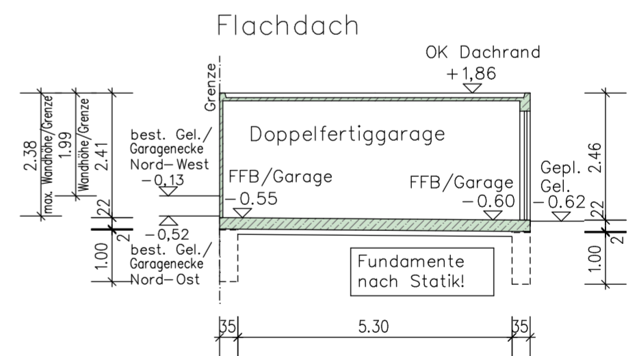
SCHNITT B-B (GARAGE)
