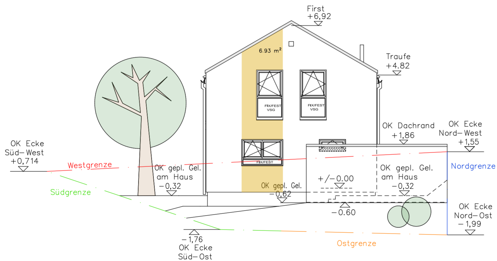
ANSICHT OST
