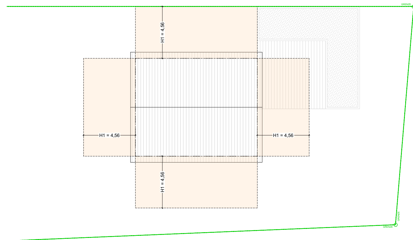
ABSTANDSFLÄCHEN m 1:200
