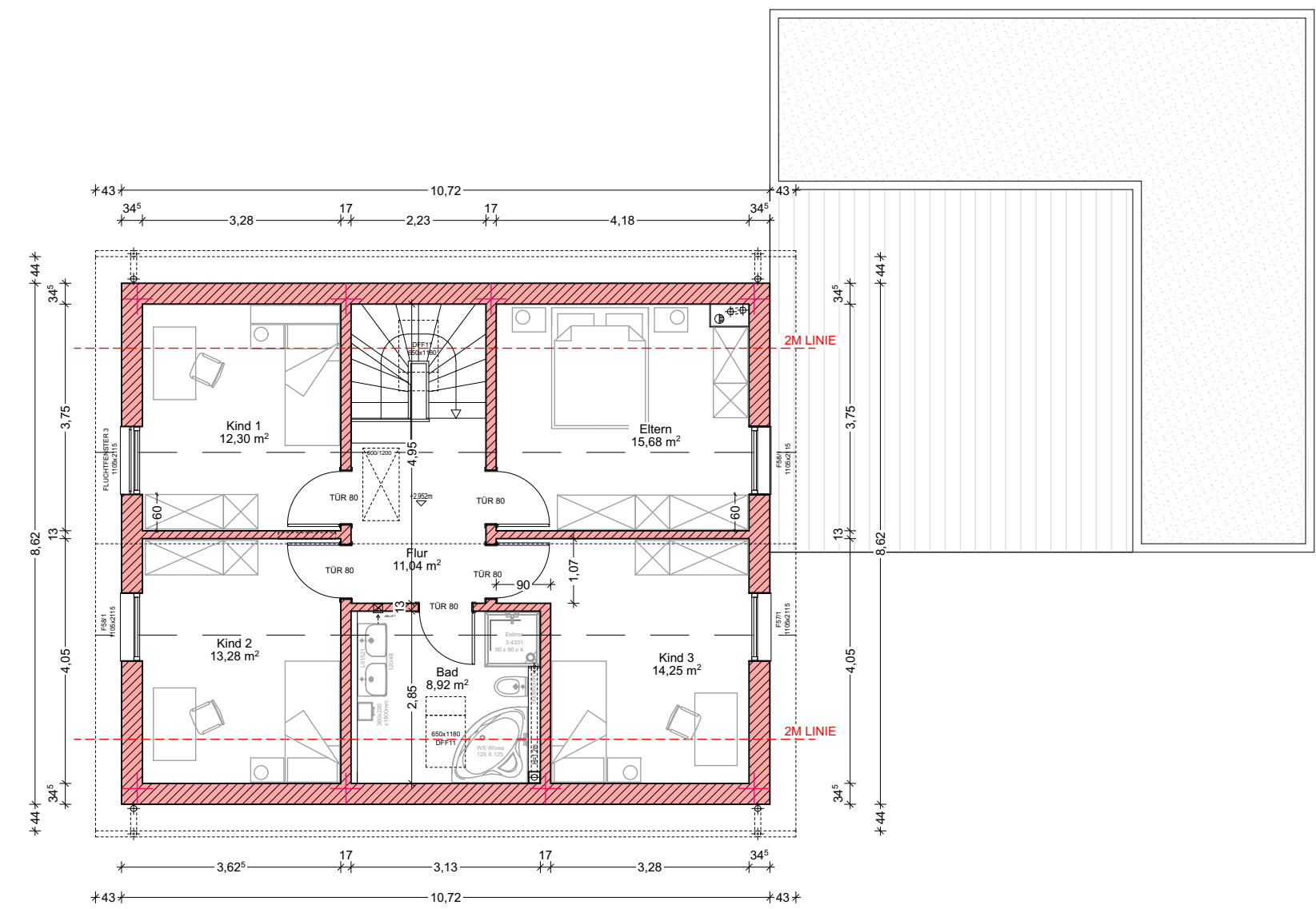
GRUNDRISS OG
