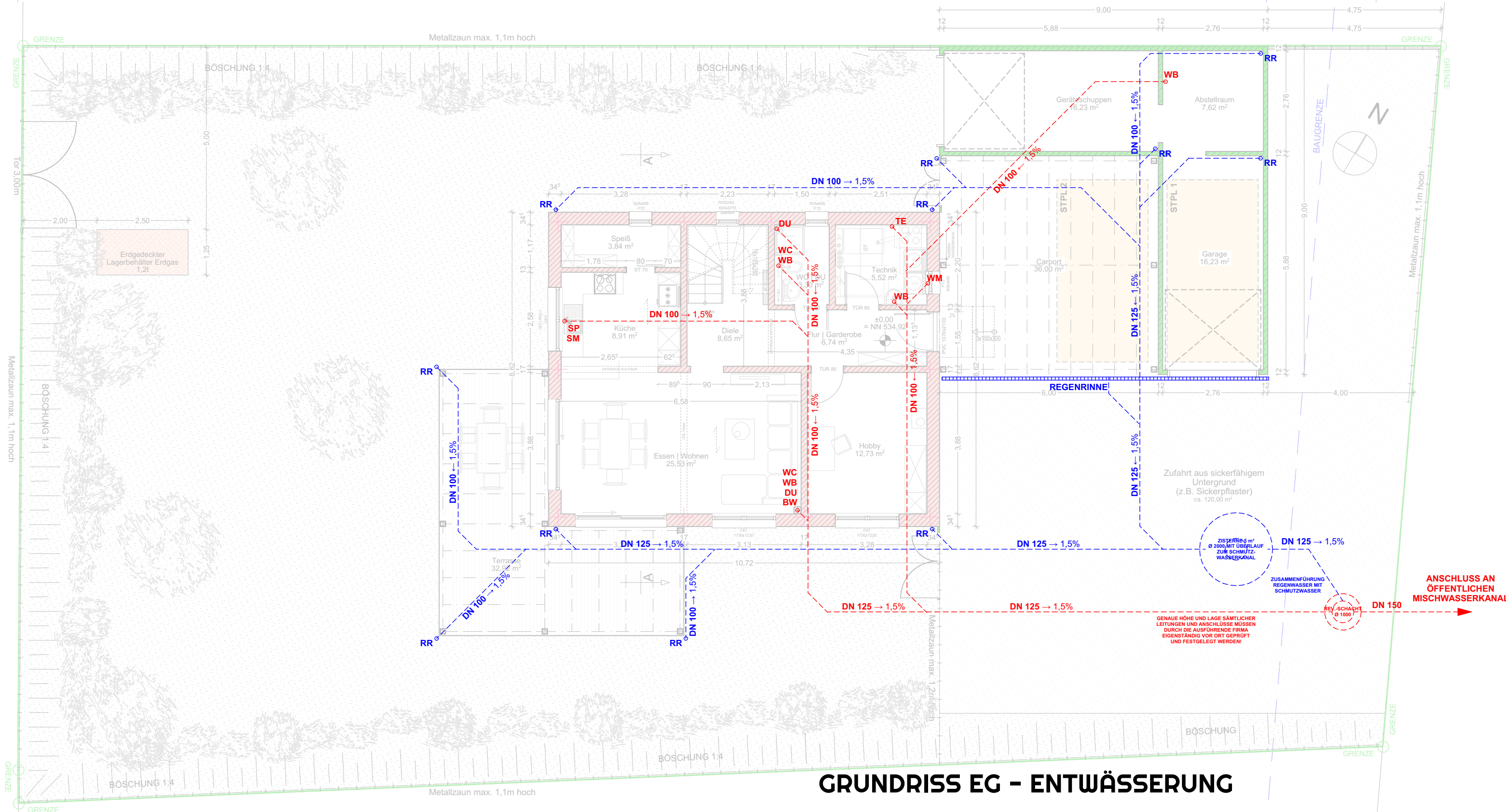
GRUNDRISS EG
