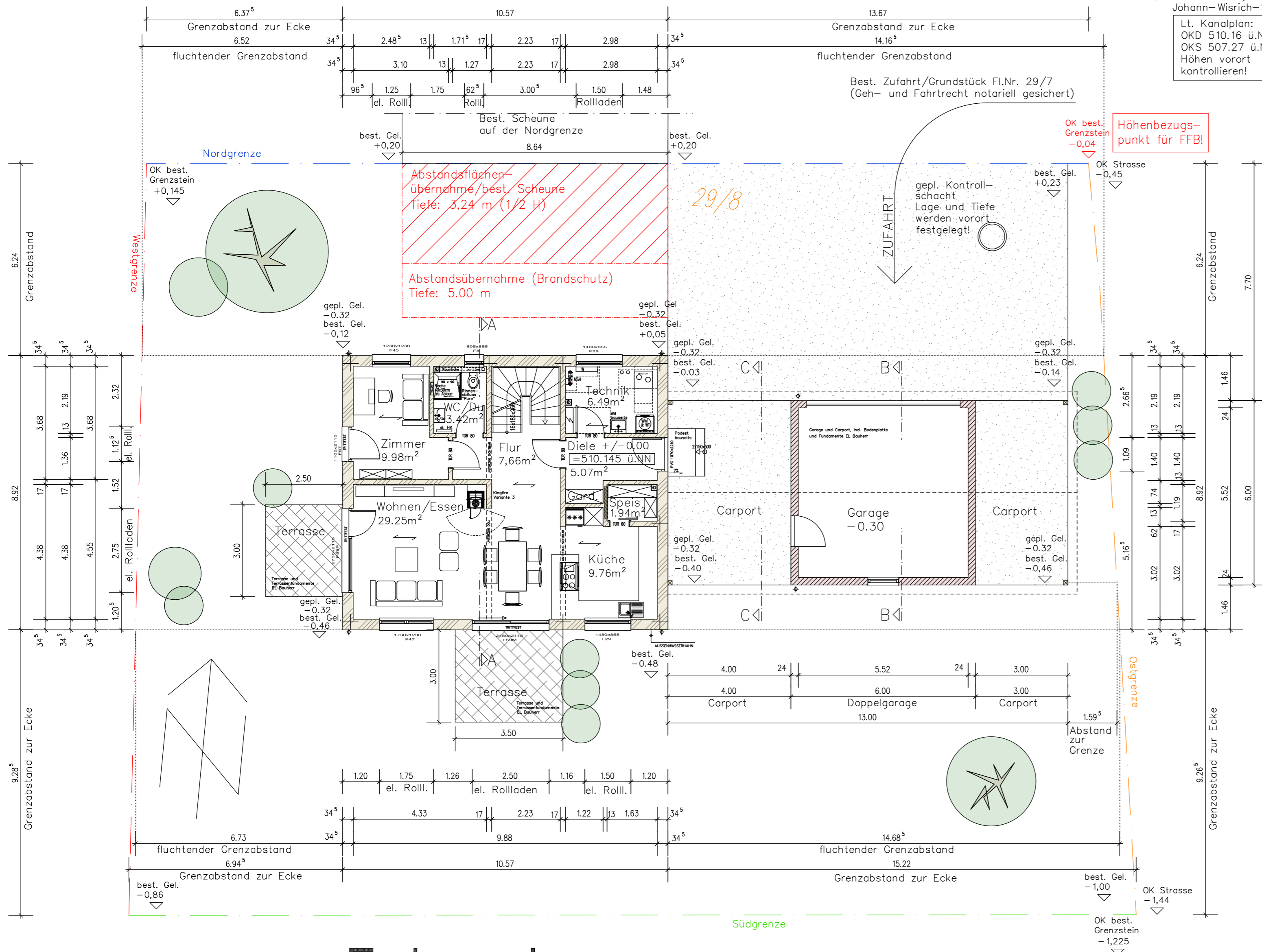
Erdgeschoss
