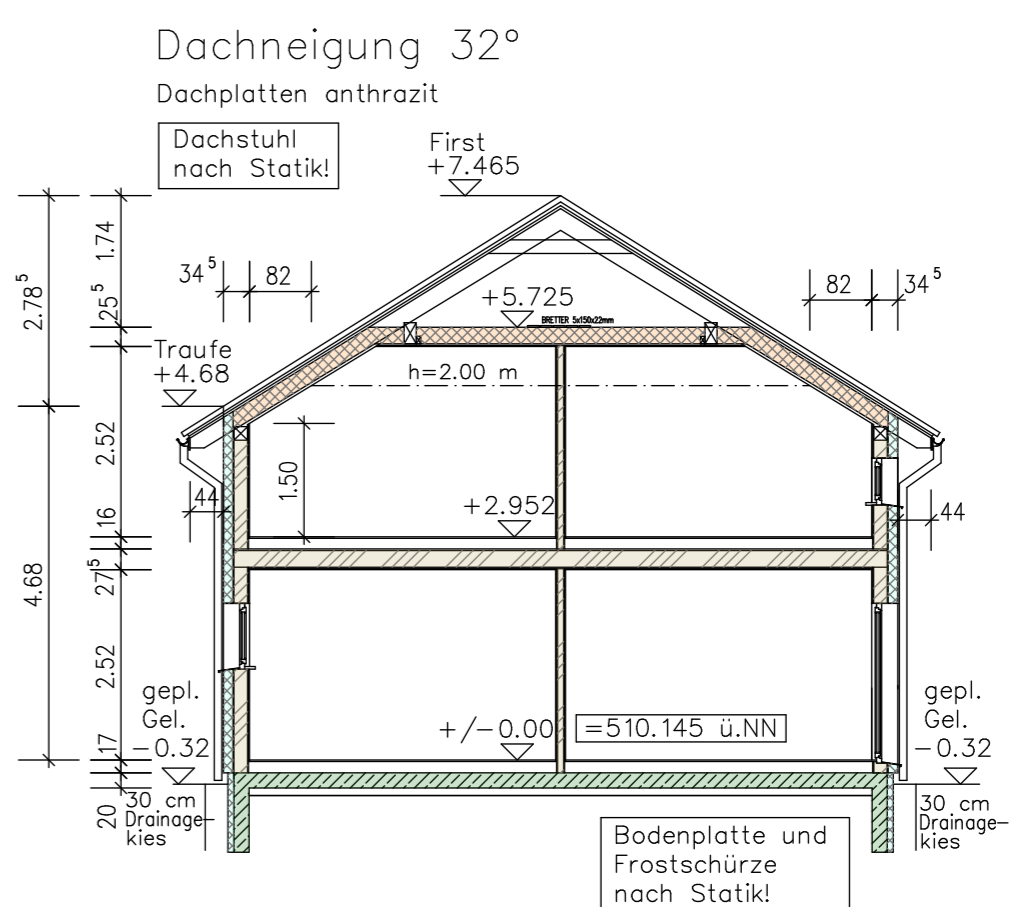
Schnitt A-A (Wohnhaus)
