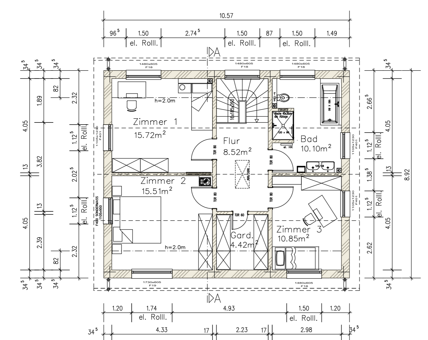
Dachgeschoss
