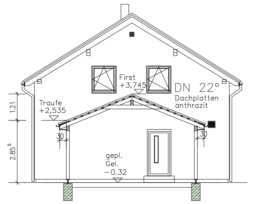
Schnitt C-C (Carport)
