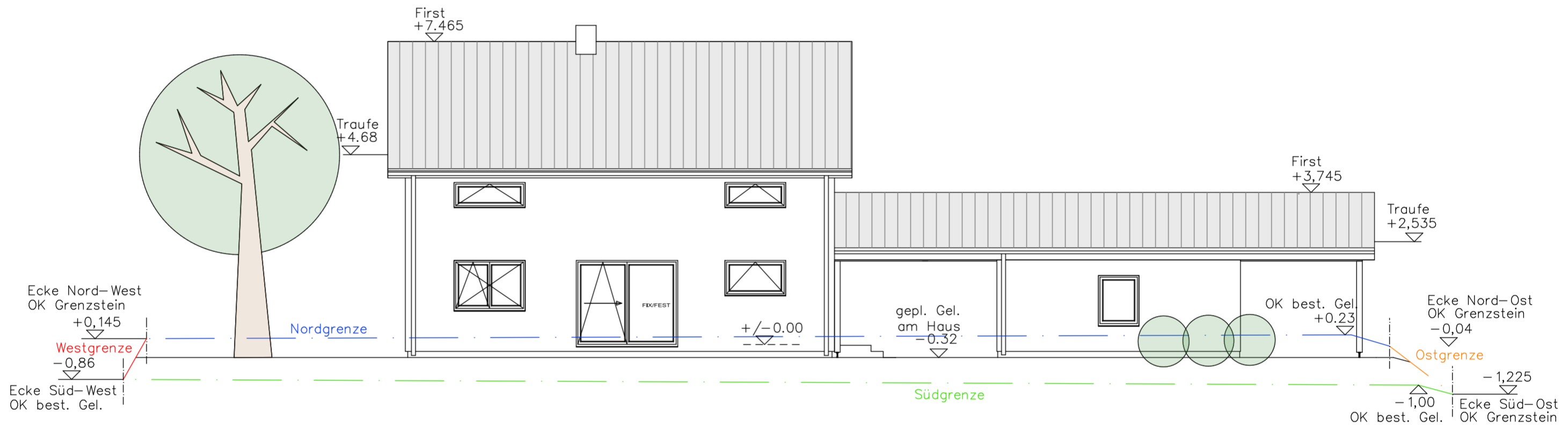
Ansicht Süd
