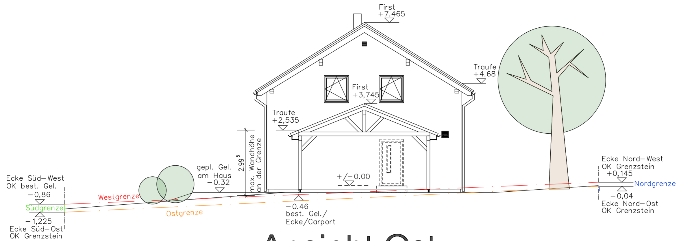
Ansicht Ost
