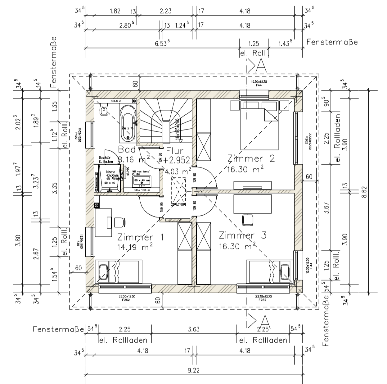
Obergeschoss
