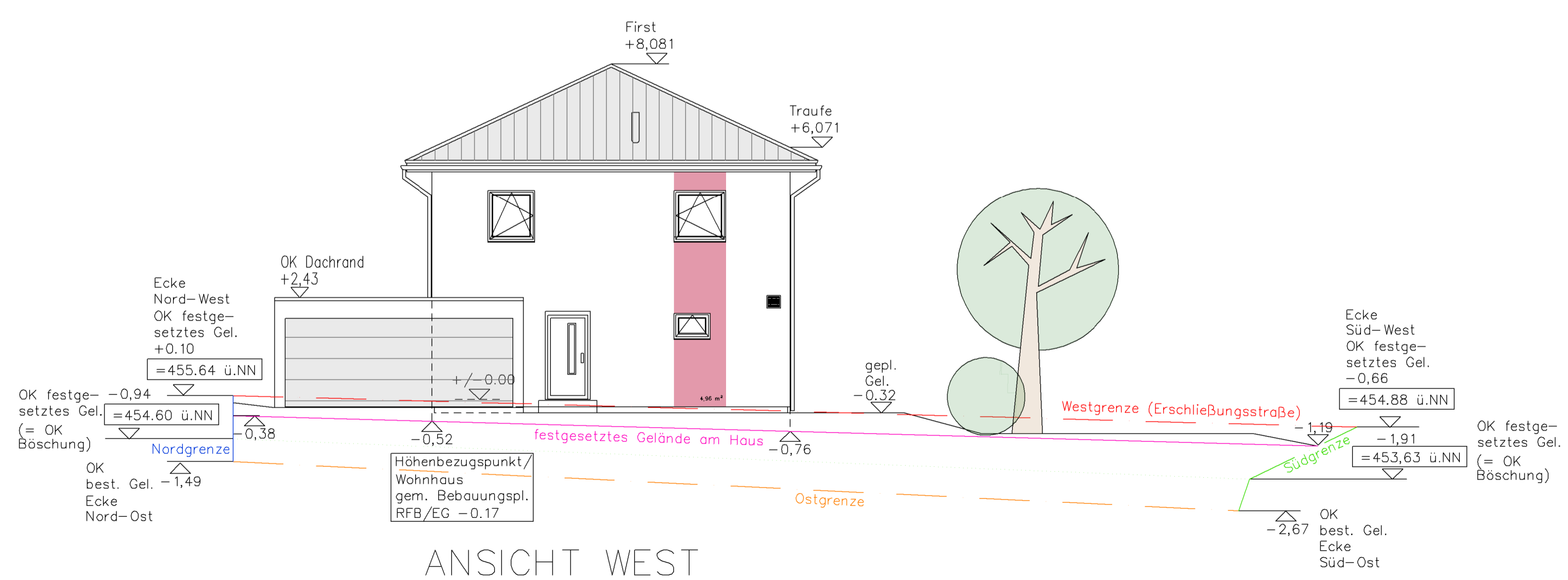
ANSICHT WEST
