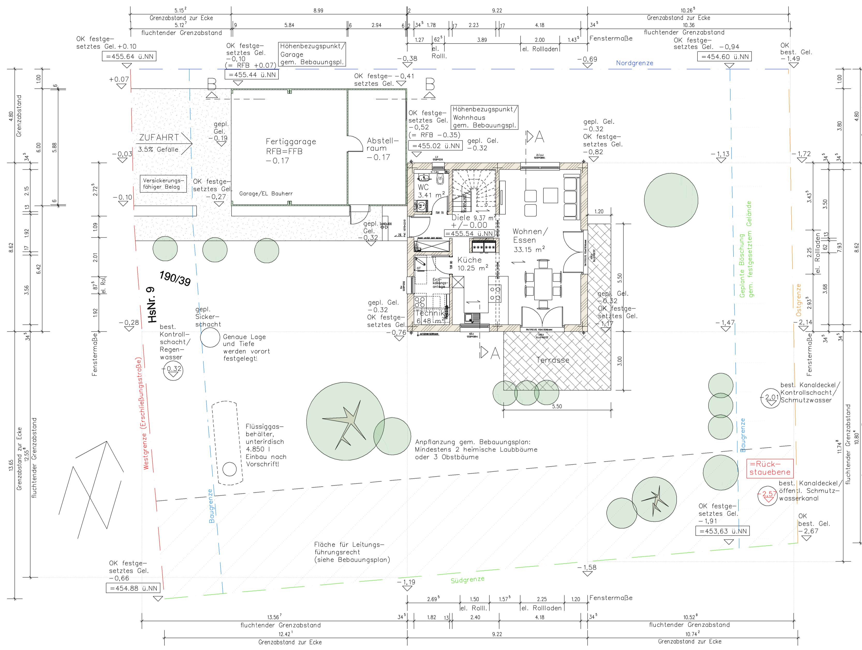
Erdgeschoss
