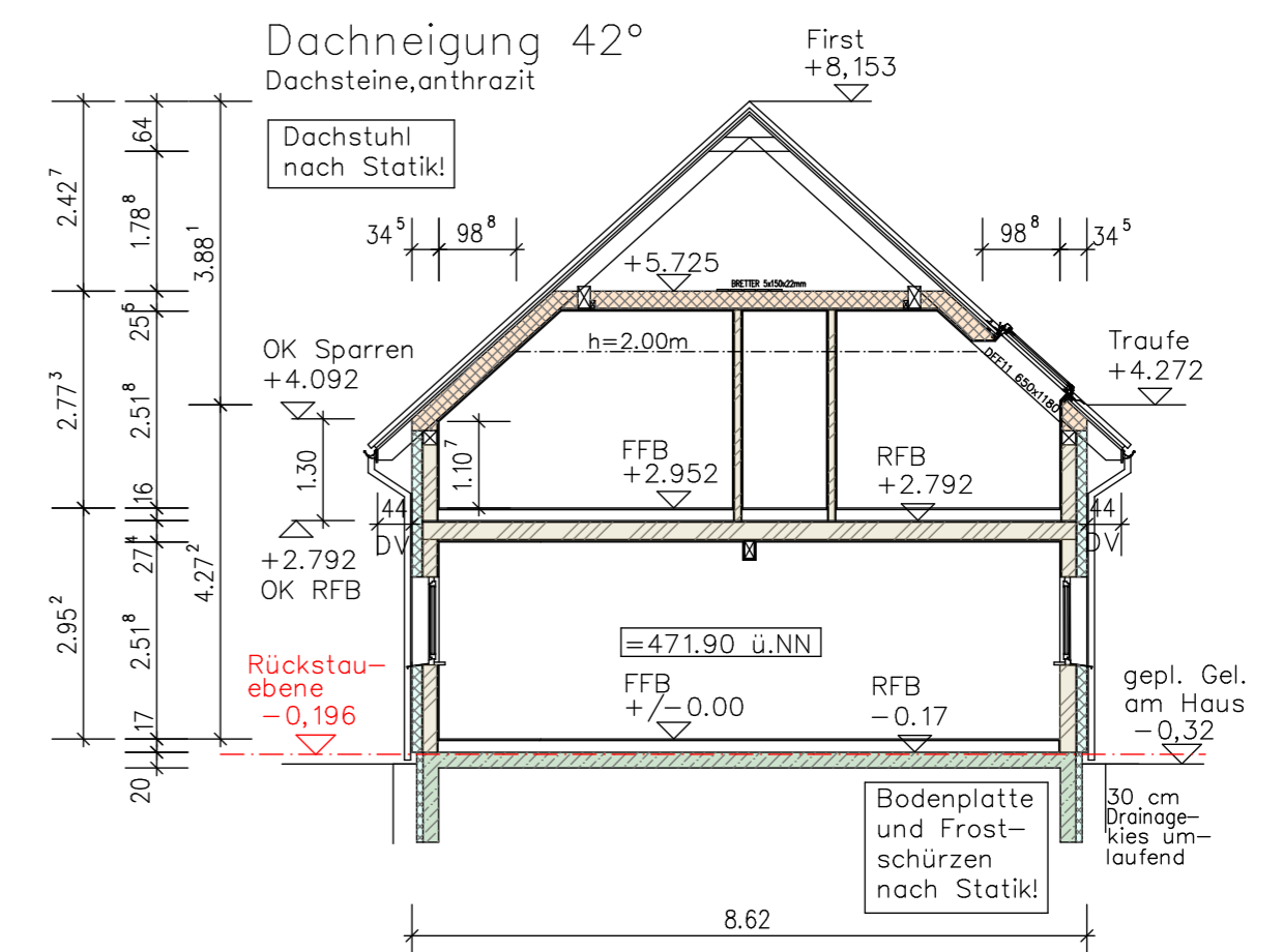
Schnitt A-A (Wohnhaus)
