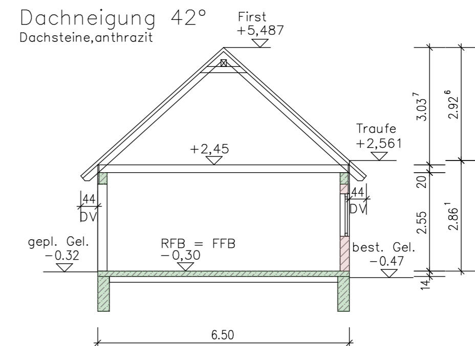
Schnitt B-B (Garage)
