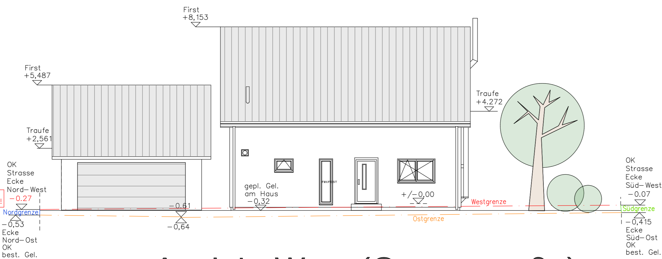
Ansicht West (Gartenstraße)
