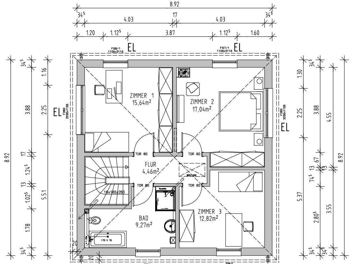
OBERGESCHOSS
