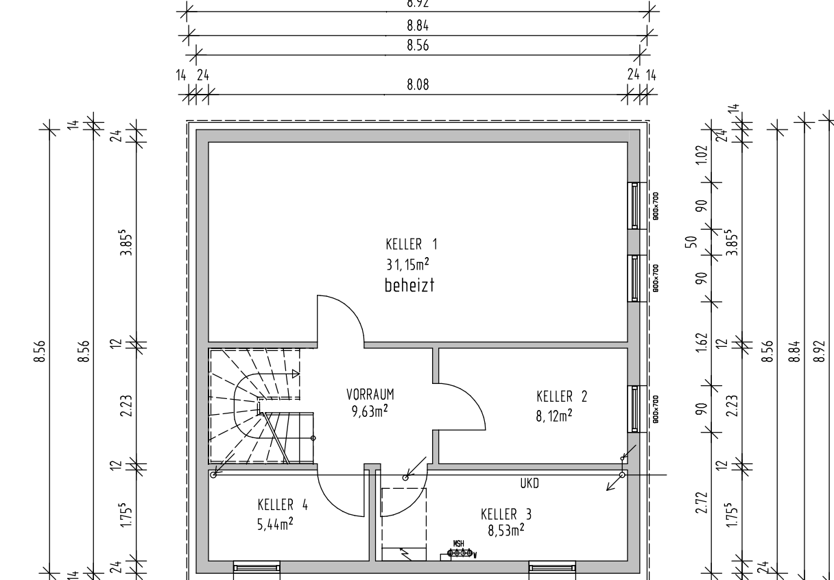
KELLERGESSCHOSS
