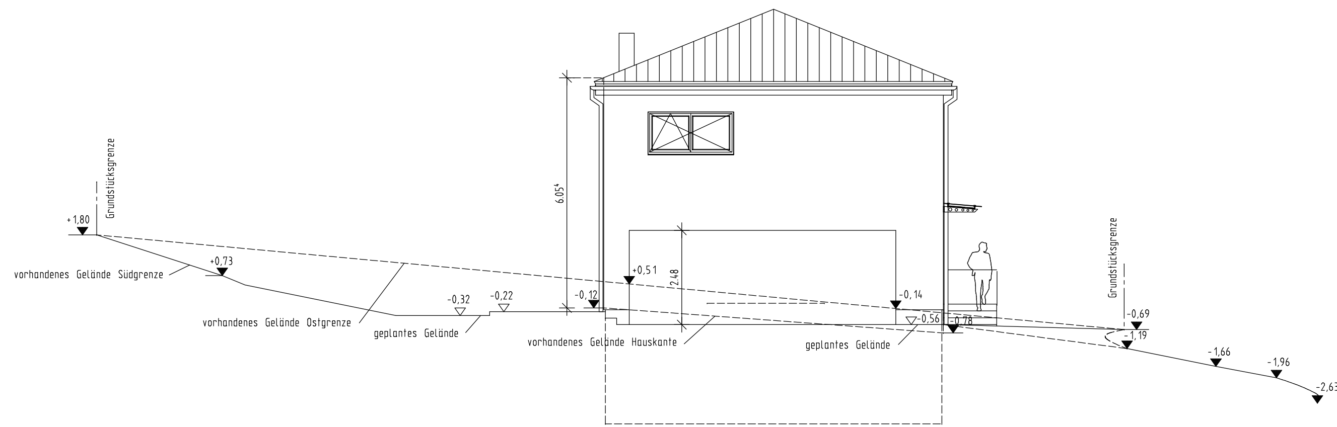
OSTANSICHT
