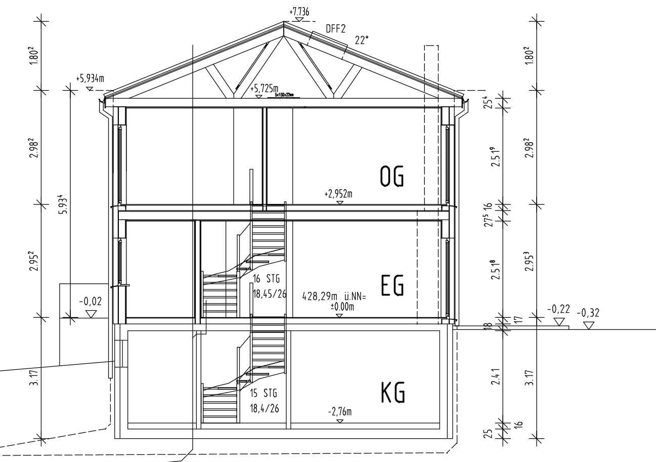
SCHNITT A-A
