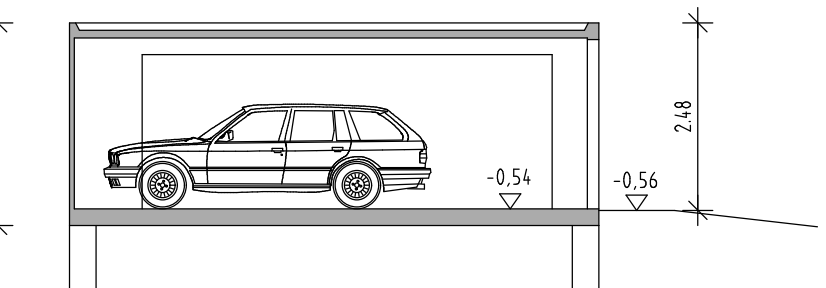
SCHNITT GARAGE
